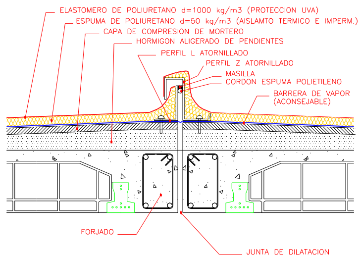
Detalle de junta de dilatación con elemento metálico
