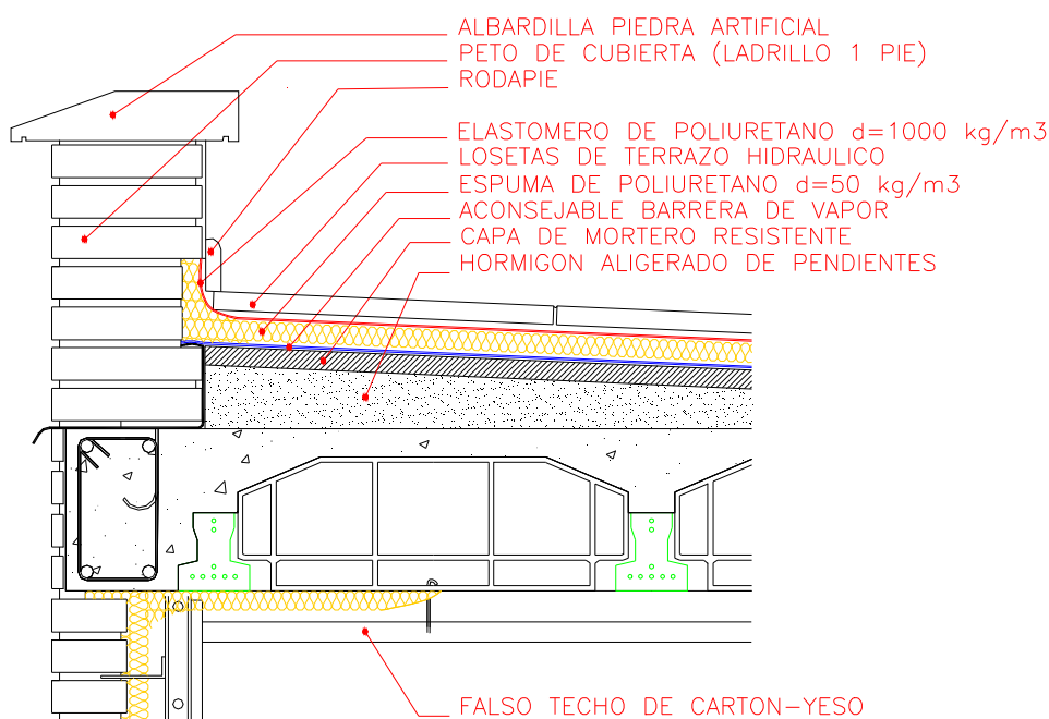
Detalle de integración de la proyección en peto de cubierta con rodapié y escuadrado de corrección de puente térmico
