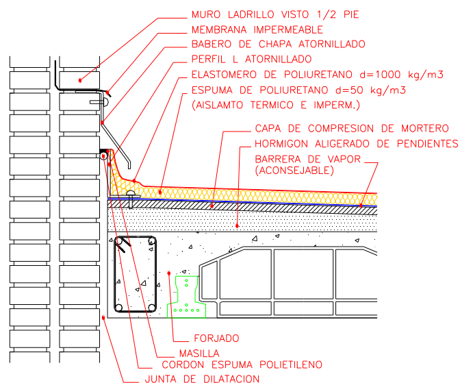
Detalle de encuentro con elemento estructural de soporte con dilatación libre
