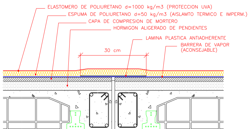
Detalle para salvar juntas de dilatación
