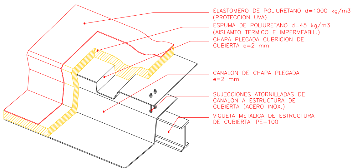
Proyección de poliuretano integrando las greca
