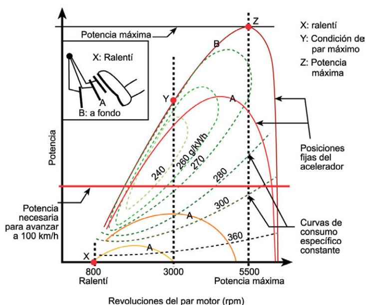
Mapa de motor de un coche moderno medio a gasolina
