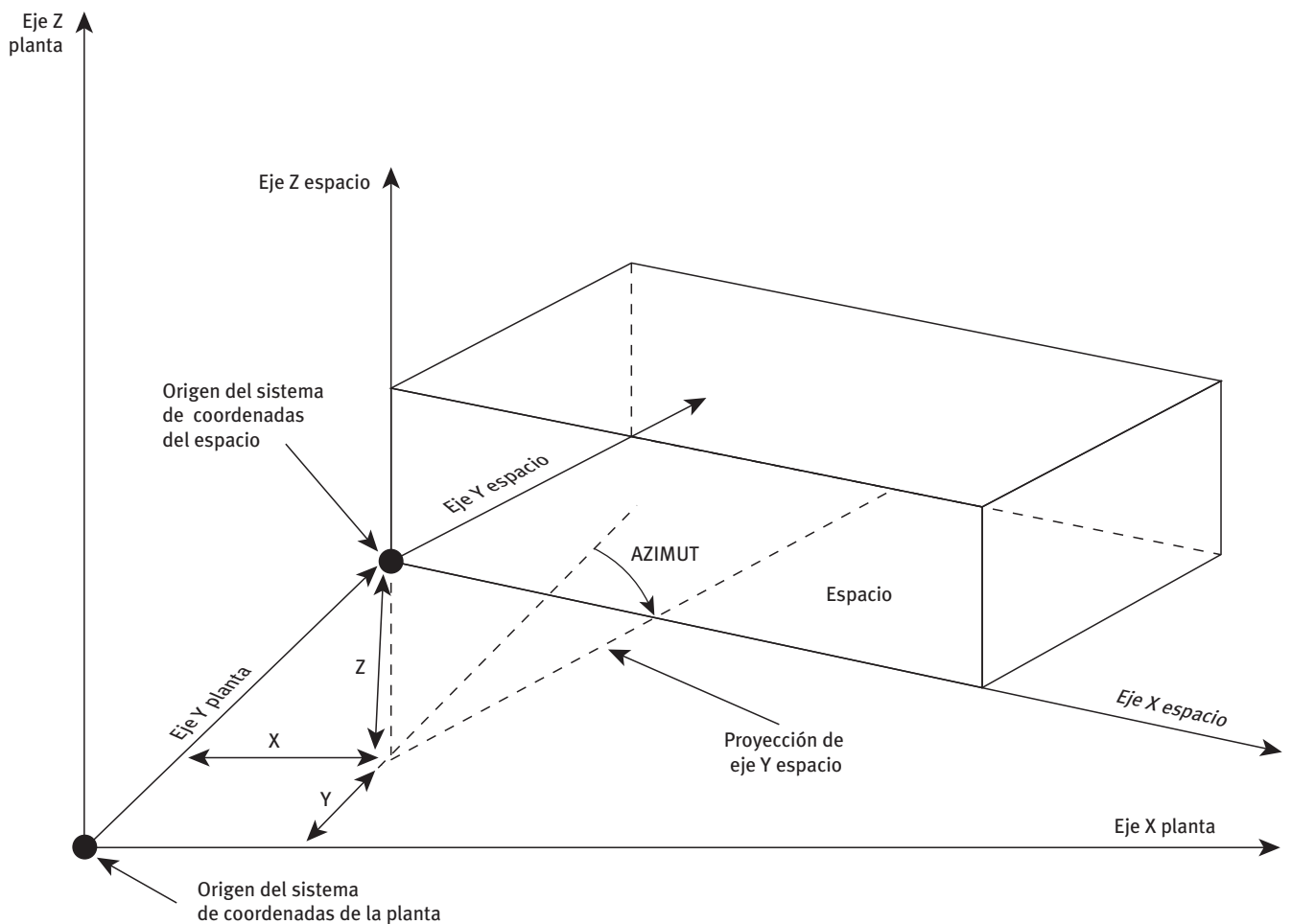
Figura 5.3 Sistema de coordenadas del ESPACIO respecto al sistema de coordenadas de la PLANTA
