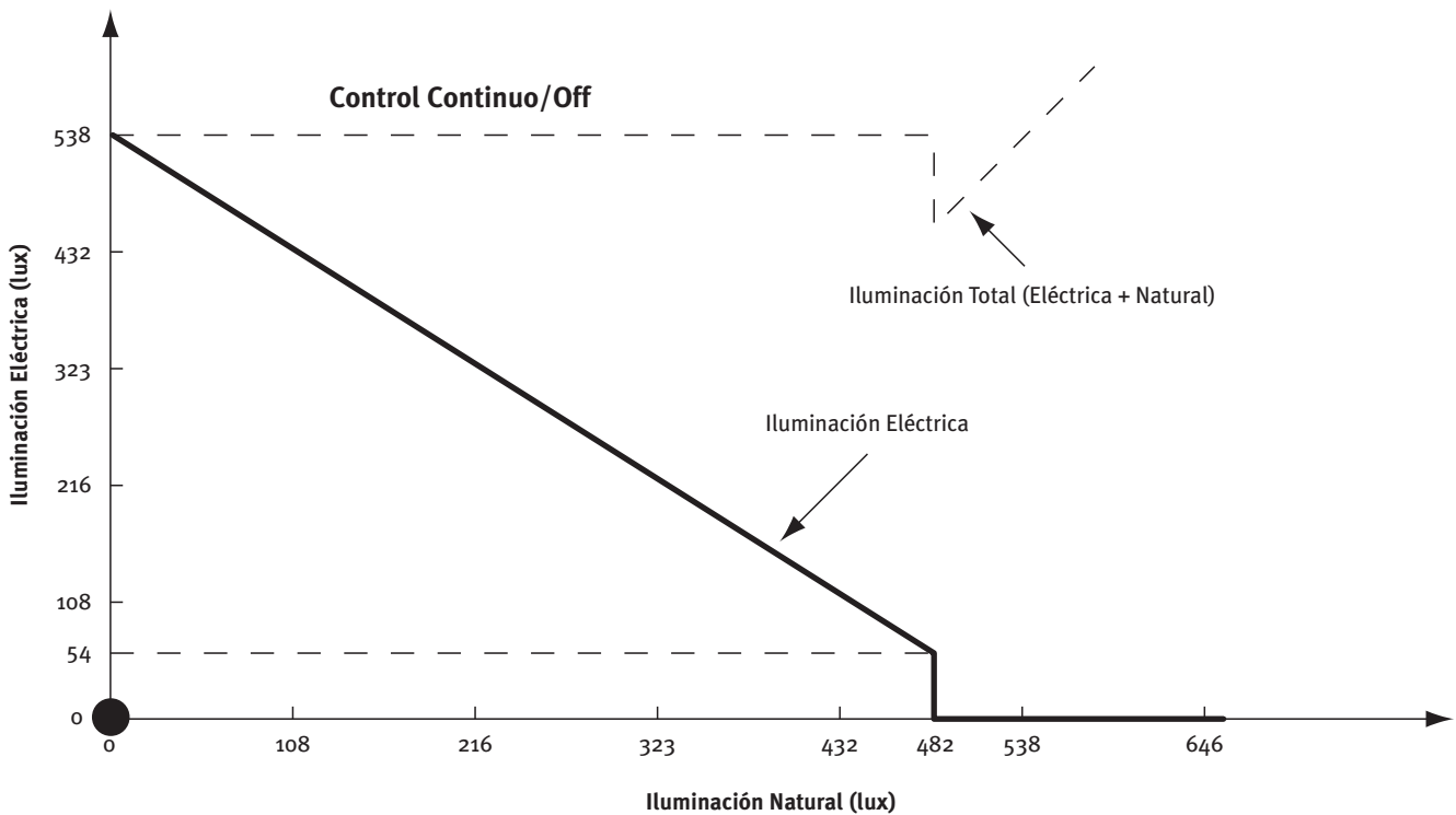
Figura 8.10 Ejemplo de control progresivo/apagado de iluminación, nivel de iluminación
