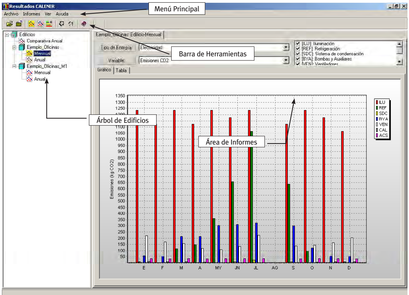
Figura 26 Pantalla principal de la Herramienta de Resultados de CALENER-GT
