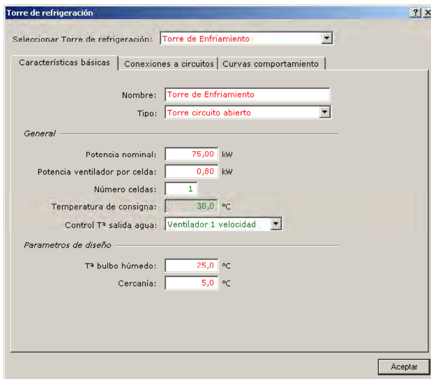
Figura 91 Diálogo de propiedades del sistema de condensación "Torre de enfriamiento", pestaña "Características básicas"
