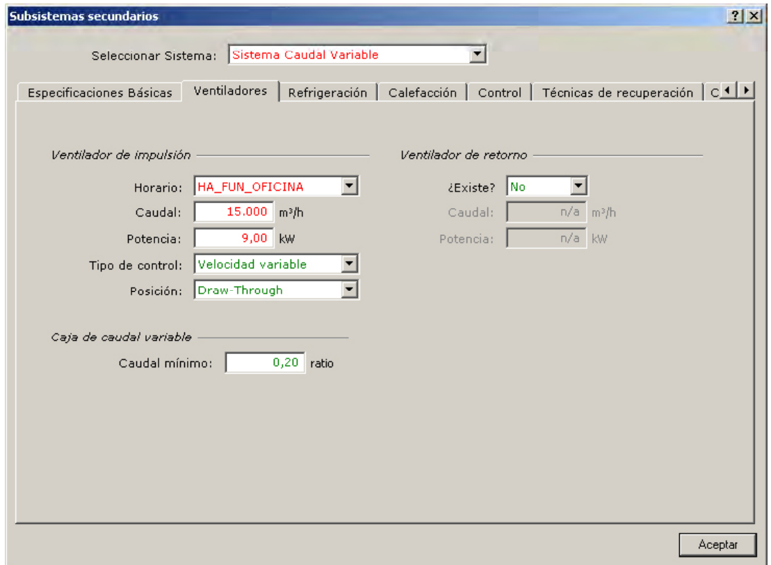
Figura 98 Diálogo de propiedades del subsistema secundario “Sistema Caudal Variable”, pestaña “Ventiladores”
