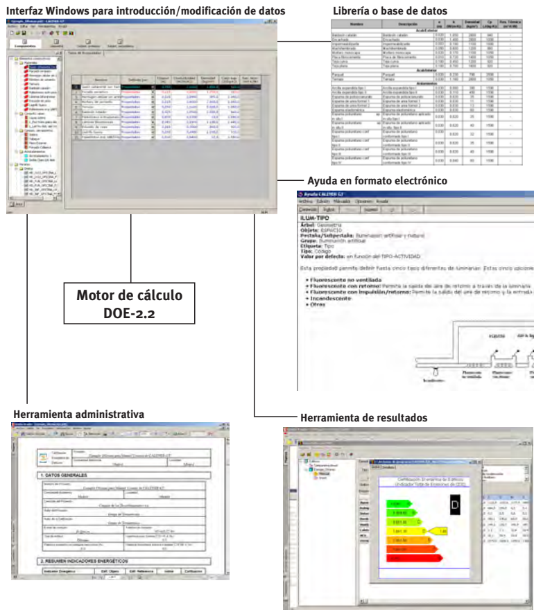
Figura 1 Herramientas incluidas en CAENER-GT
