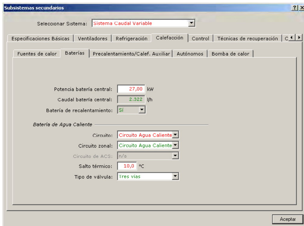
Figura 101 Diálogo de propiedades del subsistema secundario “Sistema Caudal Variable”, pestaña “Calefacción”, subpestaña “Baterías”
