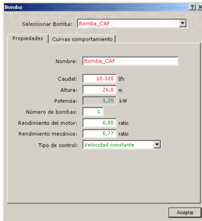
Figura 77 Diálogo de edición de propiedades de la bomba "Bomba CAF"
