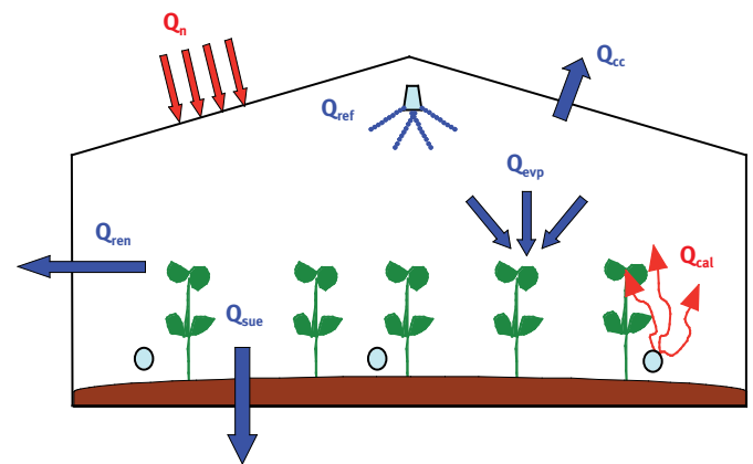
Figura 1. Balance energético en un invernadero
